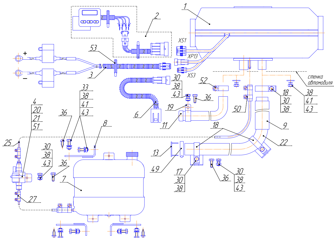
Рис.1- Схема деления воздушного отопителя на составные части.
