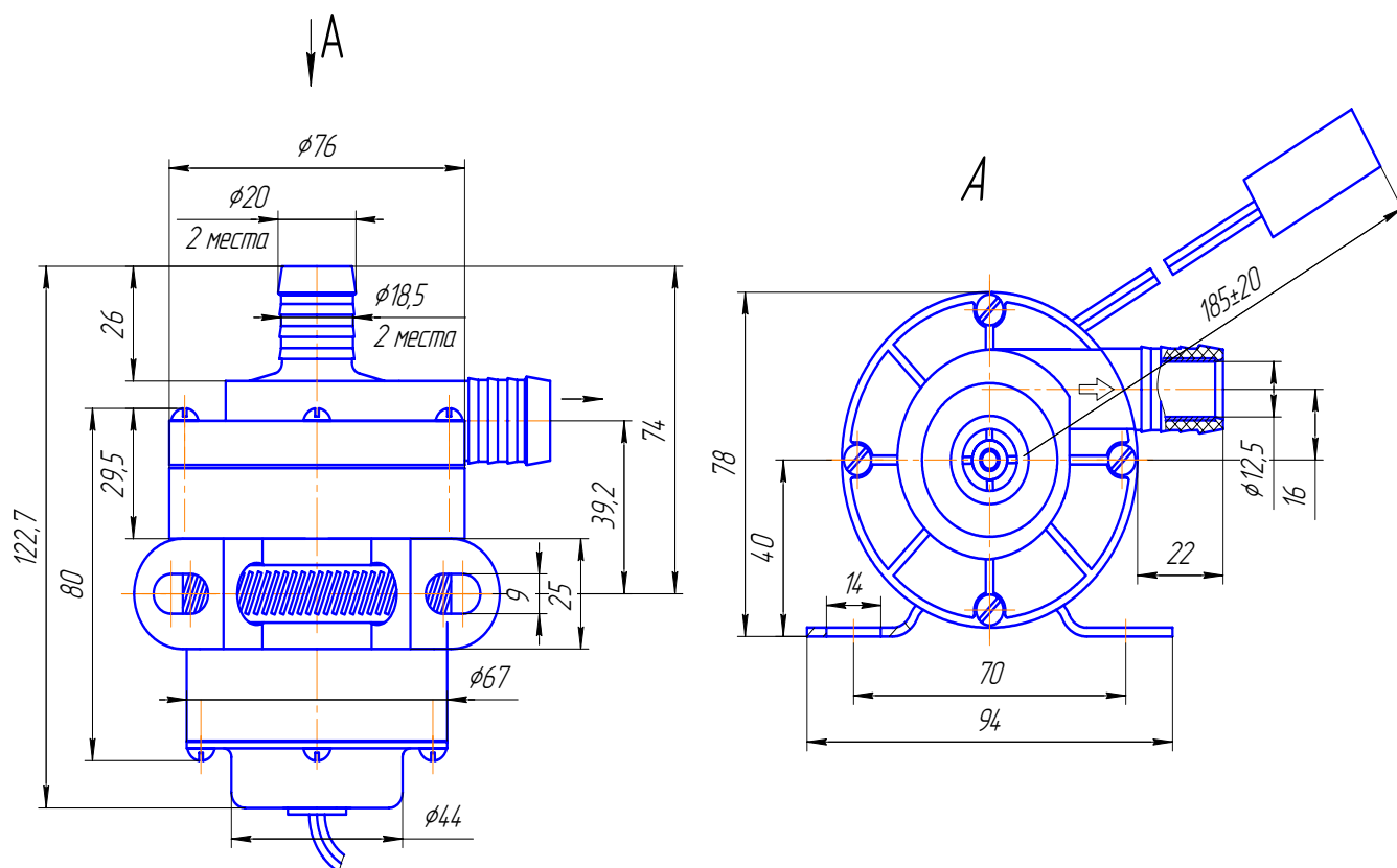
Рис.7 – Габаритные и установочные размеры П1.12В
