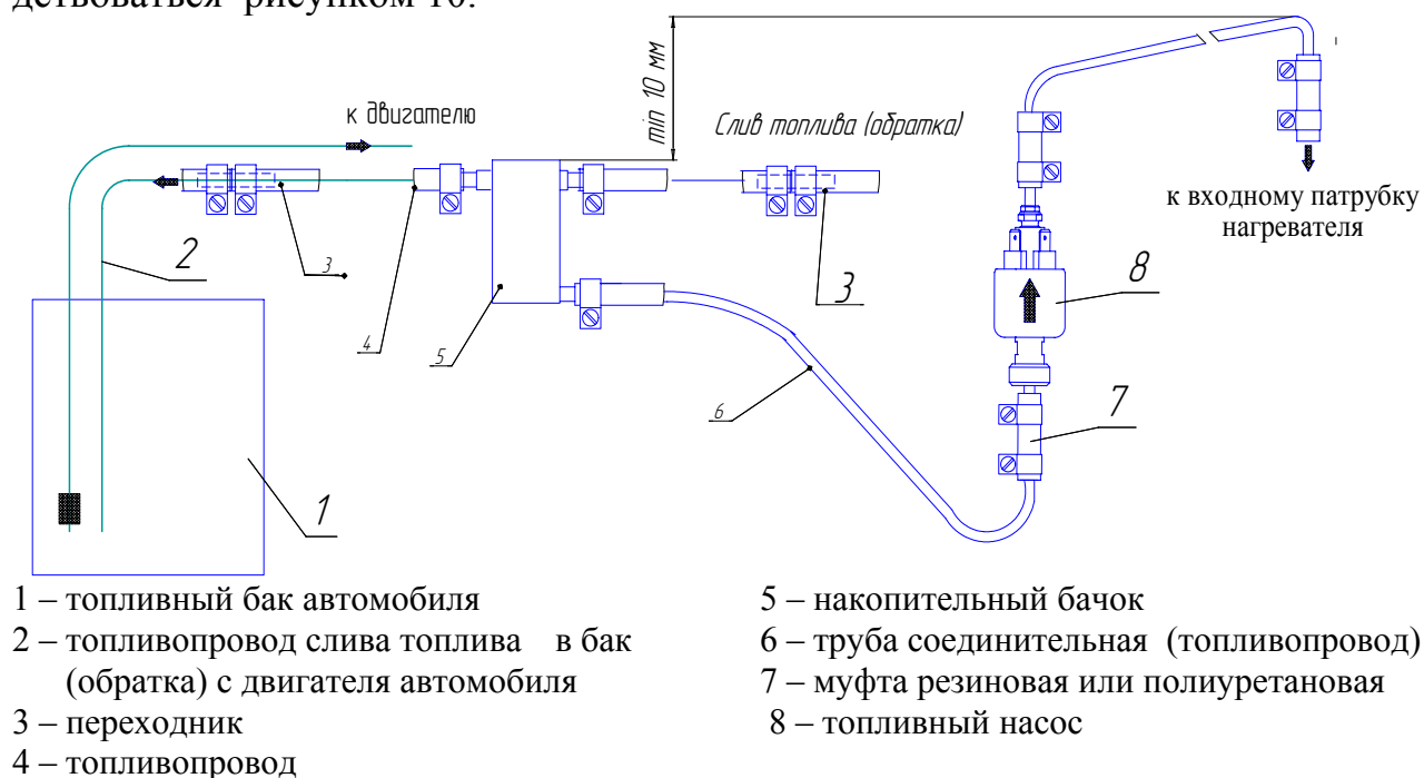
Рис.10. Схема установки накопительного бачка в магистраль слива топлива в бак (обратка) и соединение его с топливным насосом.
